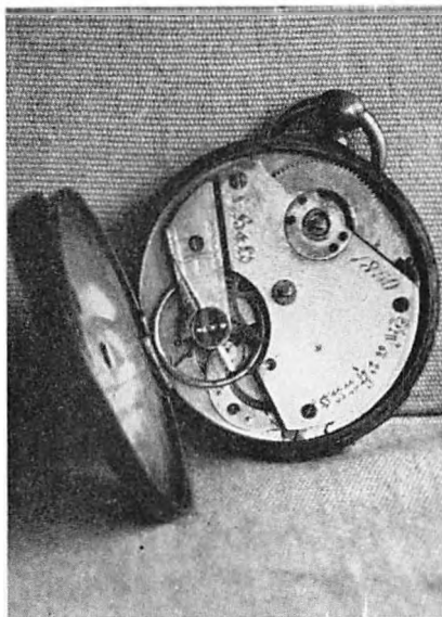
Lommeur, svendestykke af Laurits Hald 1850.
