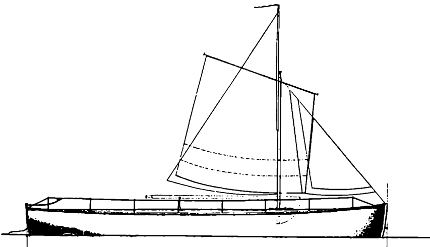
Sejltegning til en troppetransportbaad fra 1856.
