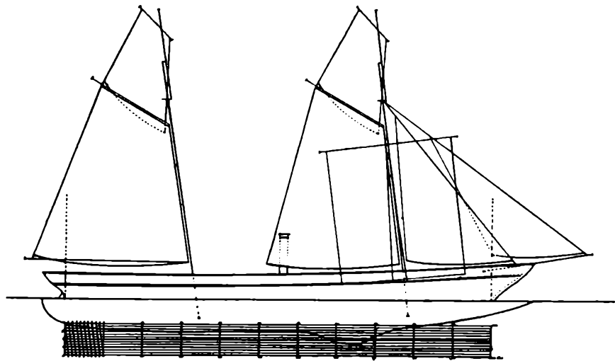
Sejltegnig til dampkanonbaaden THURA udrustet som vagerdampskib 1866—76.
