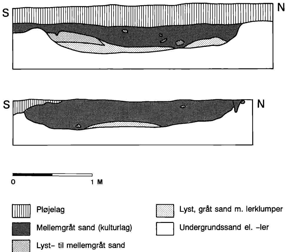
Fig. 10. Forenklet gengivelse af to profiler midt gennem hyttetomten. Den nederste profil er tegnet, efter at pløjelaget er fjernet. Yderst t.h. på tegningen ses et af pælehullerne fra hyttetomten.
