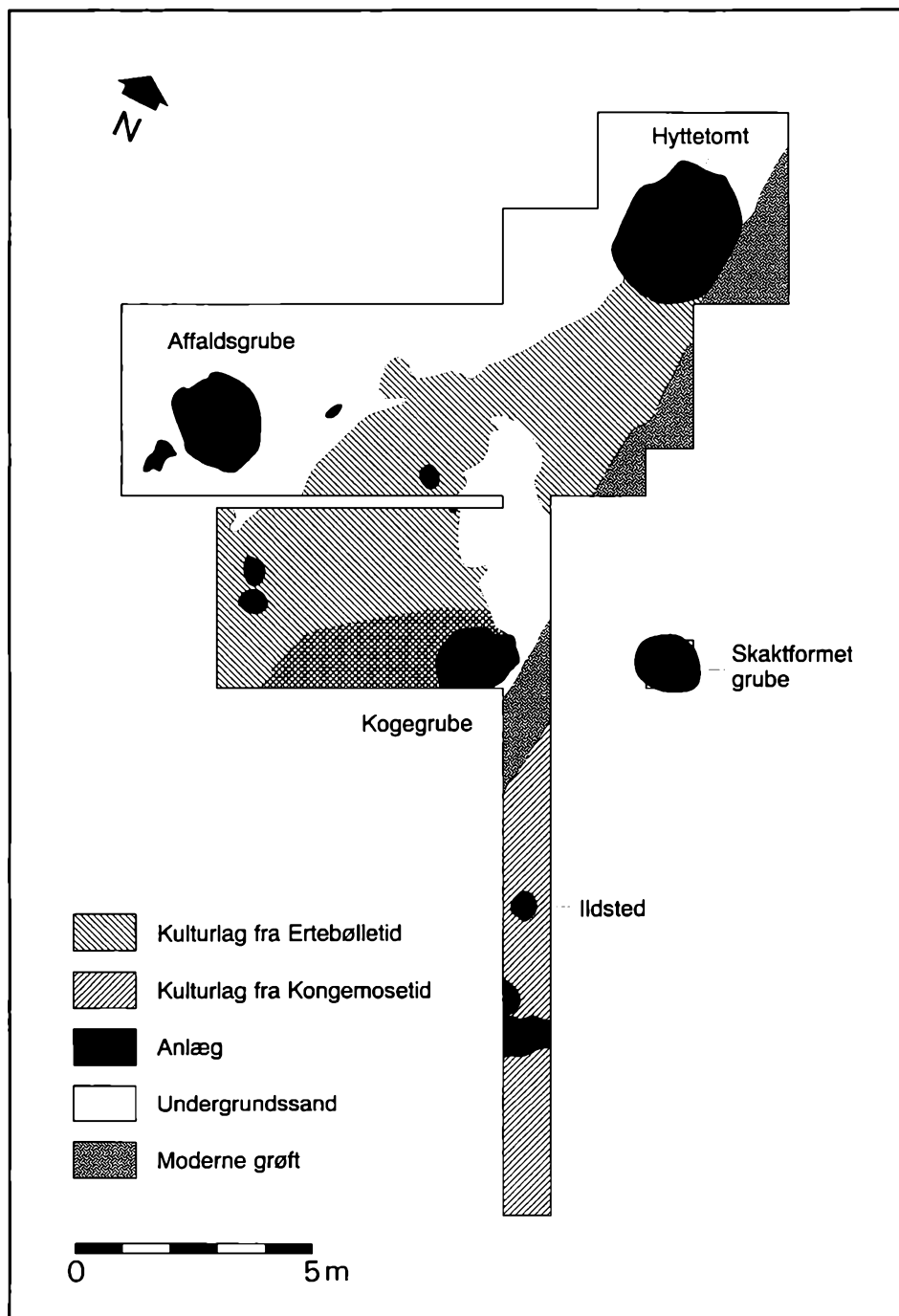
Fig. 4. Plan over udgravningen af Nivå 10.
