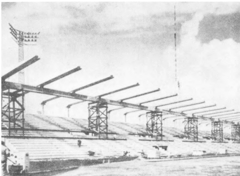
TILSKUERTRIBUNEN I GLADSAXE IDRÆTSPARK UNDER OPFØRELSEN I 1971
