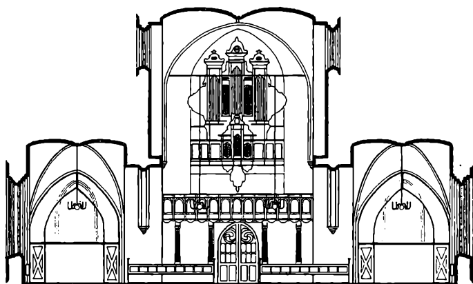
Snit i kirken set mod vest.
