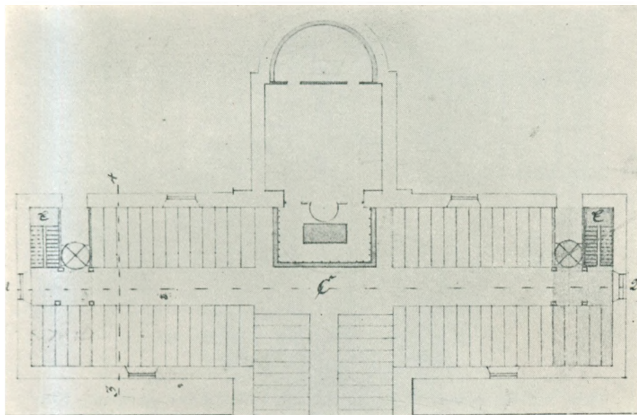
Plan over St. Jacobi Kirkes Indre efter Restaureringen 1809—12.
