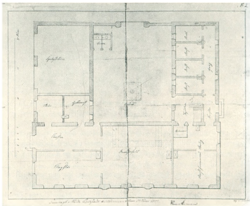
Grundplan af Varde Raadhus efter Ombygningen 1839. (Ribe Stiftamts Arkiv. Sager af forskelligt Indhold. I. 1828—48.)
