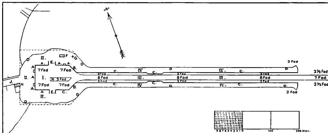
„Situations-Kort over Canalen og Havnen ved Weile, saaledes som den var ved Slutningen af Aaret 1828.“ Optaget og tegnet af Jeppe Jensen Havnefoged. I. Bassinet eller Havnen. II. Løsepladsen omkring Havnen. III. Canalen. IV. De paa begge Sider af Canalen opkastede Dæmninger. A. Bølværket omkring Bassinet. B. Tvende Stykker Pakværk. C. Pæle- eller Paskinværk. D. Simpelt Gjerde eller Fløtteværk. E. Tvende Sløbesteder. F. Havnens Materielhuus. G. Fyrstedet. H. Det nye Toldbodpakhuis med Gaard. J. Den nye Vei fra Byen til Havnen. K. Det Stykke i Bassinet, som ikke er opmudret. (Kopieret efter den originale Plan i Rigsarkivet.)
