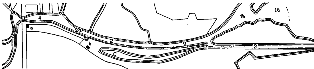
Vejle Sønderaa, opmaalt 1823—24 af Landinspektør U. Oxholm (Originalen findes i Rigsarkivet). a. „Den sydre Consumptions-Bod“. b. Havnehuus. c. „Den døde Canal“. (De vedføjede Tal angiver Vandets Dybde i Fod.)
