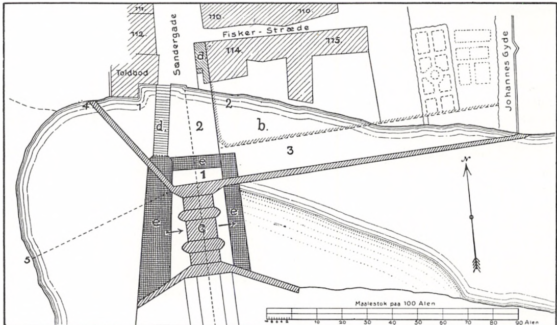
»Den sydlige Deel af Weile 1804« (Plan over Brobygningen, kopieret af C. V. Petersen efter v. Kochens Arbejds-tegning i Rigsarkivet). a) Det, som er at nedbryde af Jens Ottesens Gaard i Nr. 114, udgjør i Kvadratinhold 82 Alen. b) Det Vederlæg, som kan gives af den opfyldende Plads, udgjør i Kvadratinhold 624 Alen. c) Den nye Bro, som er under Arbejde. d) Den gamle Bro. e) Dæmningen omkring Broen. — Den Plads, som er bestemt til at opfyldes efter 1, 2 og 3, er anslaaet til 1450 Kvadratalen.
