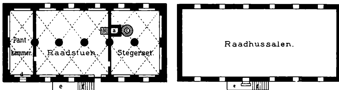
Plan af Veile Kloster-Raadhus. 1631. Til venstre: Nederste Stokværk; til højre: Øverste Stokværk.
