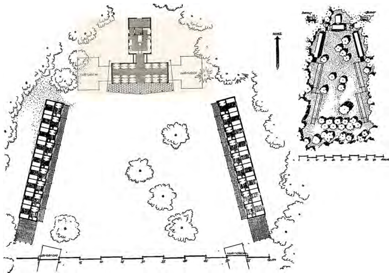
'Skitse af Bebyggelsen. Til venstre den vestlige Gæstelænge med sydvendt Pergola for Enden af Længen. I Baggrunden ses Hovedhuset med overdækket Siddeplads mod Syd, og yderst til højre skimtes den østlige Gæstelænge mellem Træerne.
