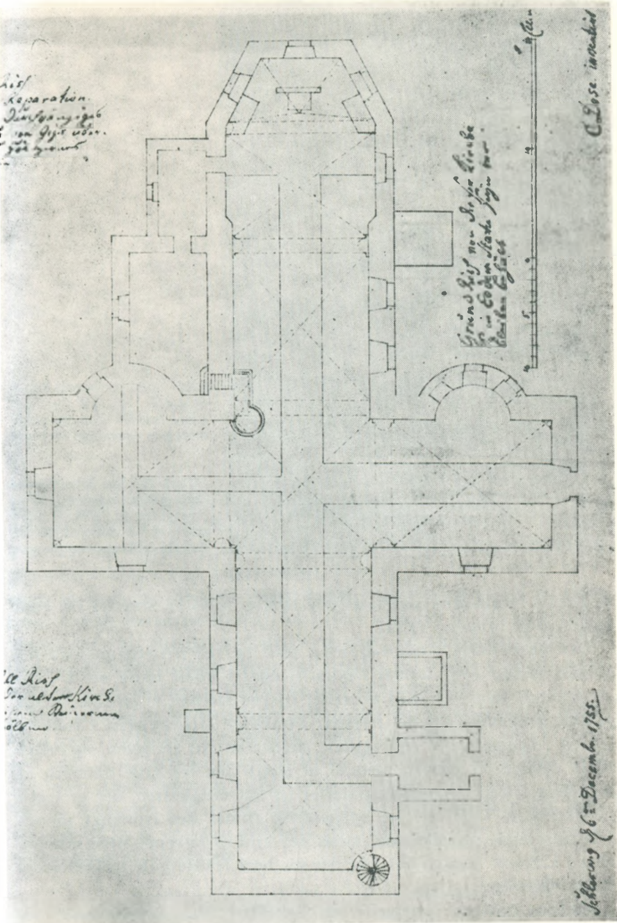
Grundplan af Skt. Nikolai kirke. Opmålt af C. Dose 1755.
