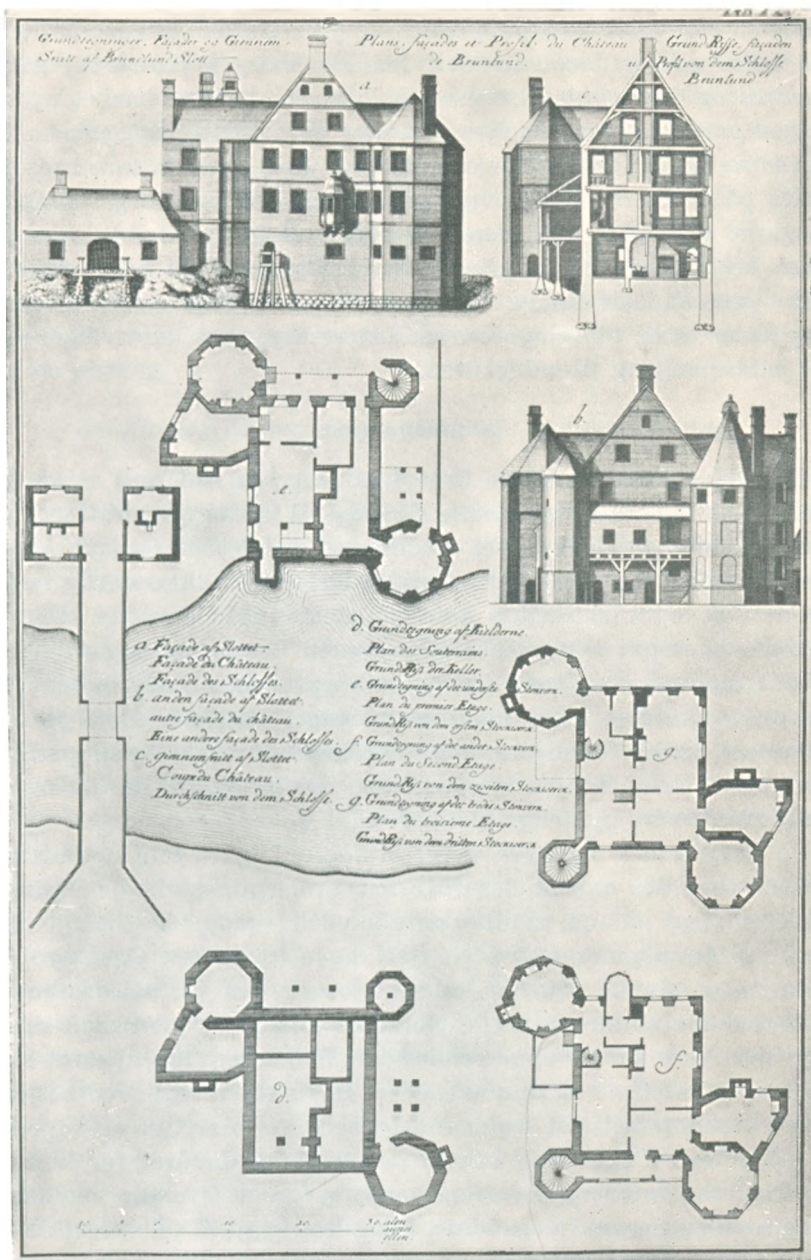
Brundlund slot. Facader, snit og grundplaner, 1749.
