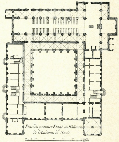
Plan af stueetagen, Sorø Akademi ca. 1749.
