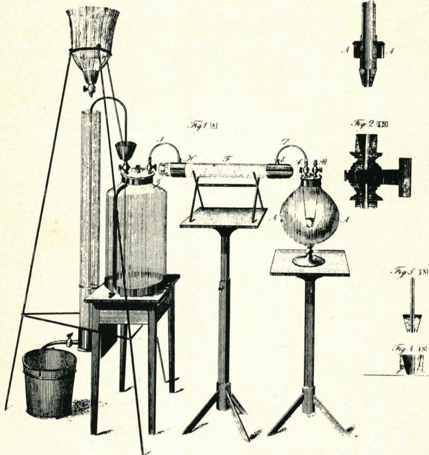
Opstilling til undersøgelse af Fosfors forbrænding. Hollandsk. Højde ca. 2 m, længde ca. 2 m. Kobberstik fra Hauchs bog »Det fysiske Cabinet« 1836.
