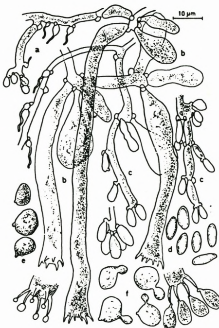
Fig. 1. Syzygospora sorana. a. Haustoria; b. Basidia; c. Conidiophores; d. Conidia; e. Spores; f. Spores, producing blastoconidia.
