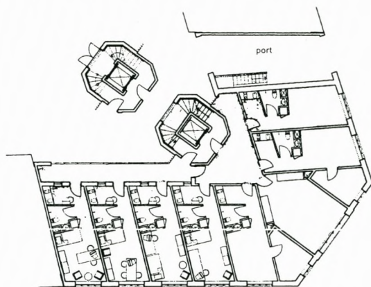
Stueplan
