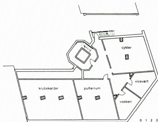
Kælderplan
