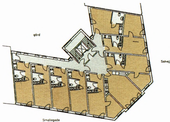
Etageplan
