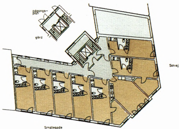
Stueetage
