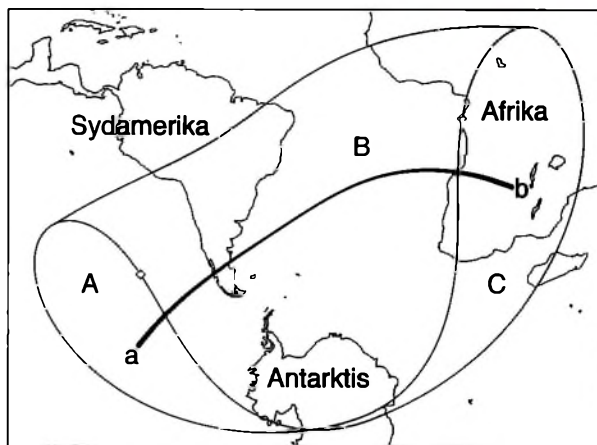
Ringformet solformørkelse 26. februar 2017
