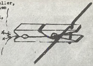
Tændingsmekanisme fra sabotagens barndom. Tøjklæmmen holdtes ved hjælp af en snor åben, indtil f. eks. et tog kørte over den. Når klæmmen smækkede sammen, sluttedes en elektrisk strøm og eksplosionen udløstes.
