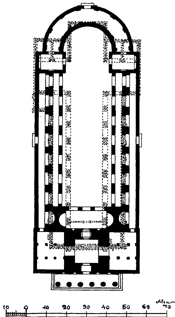
Plan af Vor Frue Kirke i Kjøbenhavn og Sorø Klosterkirke (punkteret).
