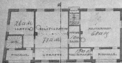
STUEN.
