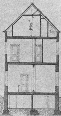
PROFIL EFTER A-B.
