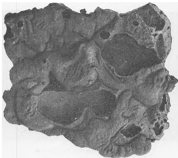
Slagge fra Forekomsten i Skoven Nyvænge, V. Aaby Sogn Fra 14. Aarh. \frac{1}{2} Størrelse. (Gruberne skyldes Luftblærer i den tyndtflydende Slaggemasse). Fra »Fynsk Hjemstavne».
