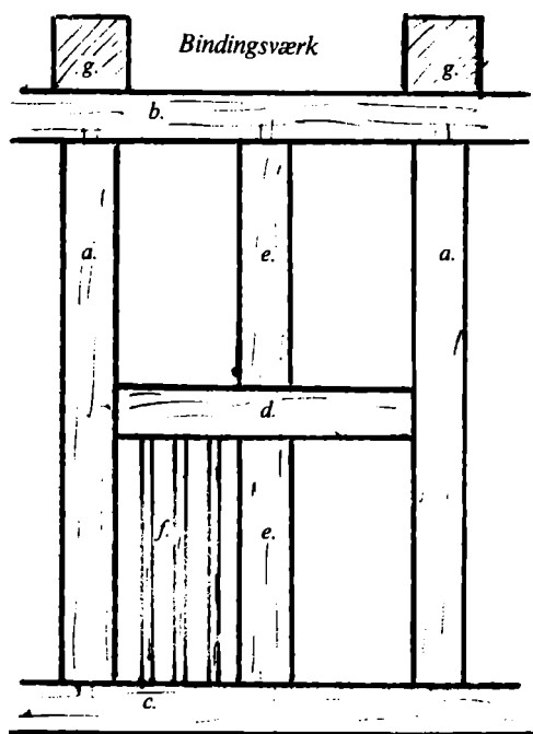
a. stænger eller stolper; b. loftsrem; c. fodrem; d. løsholt; e. dokter; f. spoler, om hvilke vidjer eller halm svøbtes i kurvestetning. Derpå klaskedes så det våde ler; g. loftsbjælker.
