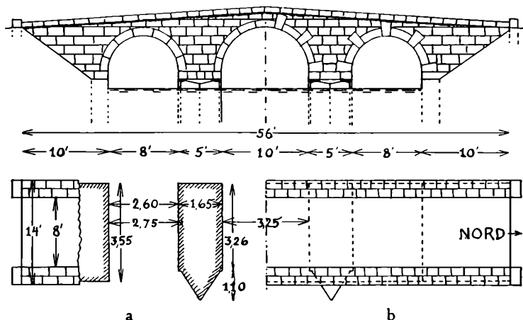
Rekonstruktion af Løvel bro 1:200. 1)
