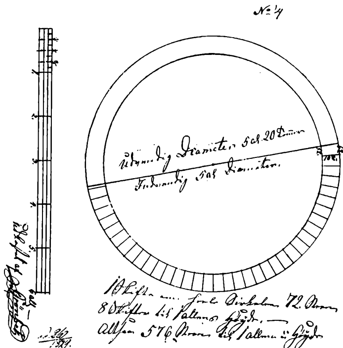
Skitse til stenenes anbringelse i skakten (bilag til Lhs. indkomne sager 260/1829).
