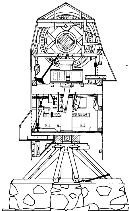
Skematisk tegning af stubmølle.
