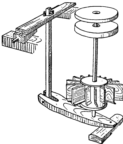
Skematisk tegning af "Letteværk" fra en sqvatmølle fra Halland.
