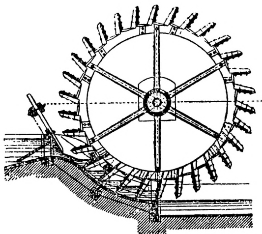
Skematisk tegning af underfaldshjul.
