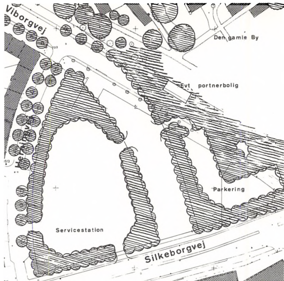
Plan over trekantområdets opdeling efter bestemmelserne i Lokalplan nr. 50. Til højre ligger område I: parkanlæg og parkering i tilknytning til Købstadmuseet »Den gamle By«. I midten område II: den regulerede Viborgvej, der løber vinkelret ind på Silkeborgvej. Til venstre område III: servicestation.
