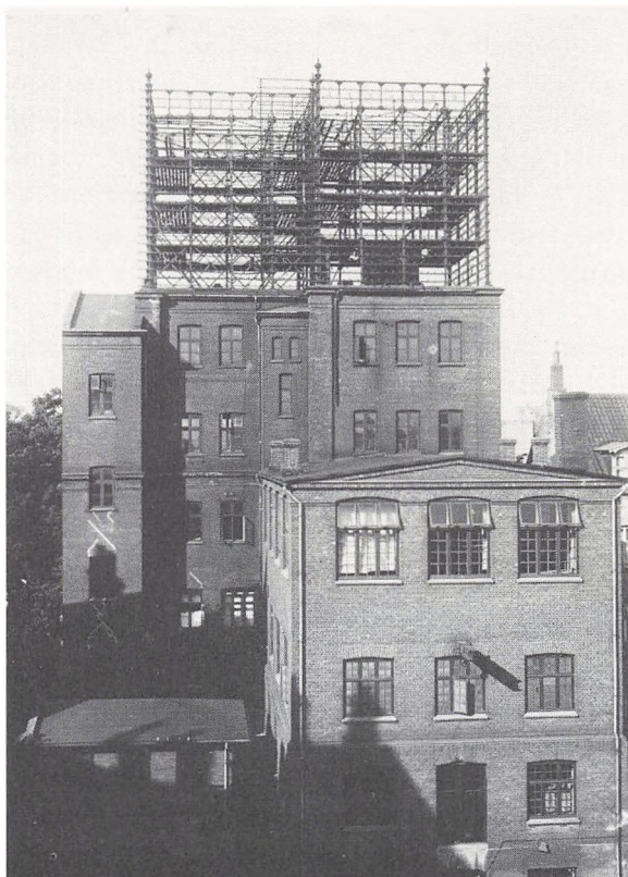
Der skulle en solid bygning til at bære Jydsk Telefons centraltårn, der lå bag Søndergade 4-6. Forbindelserne til abonnenterne gik nemlig over det store ståltårn øverst på bygningen. Tårnet blev flere gange gjort større ved påsætning af nye etager. Da det hele blev nedtaget i 1923 vejede det ca. 500 tons. Billedet er fra kort før nedtagningen. Den gamle tårns funktioner blev overtaget af jordkabler. (Foto i Lokalhistorisk Samling)
