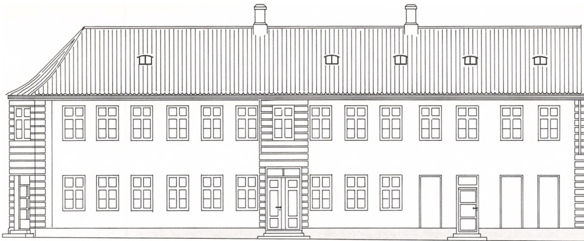
Tegning af facaden mod Immervad af Statsanstalten for Livsforsikrings nyrestaurerede bygning. Huset er fra 1808, men facaden er ført tilbage til det udseende, som bygningen fik ved en ombygning i 1843.
