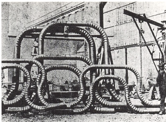
Her ses et lille udvalg af de ekspansionsbøjninger, der anbringes for hver 60-70 meter i fjernvarmenettet. Bemærk folderne på rørene, der skal optage varmeudvidelsen, der kan være op til 10 cm pr. 100 meter rør.
