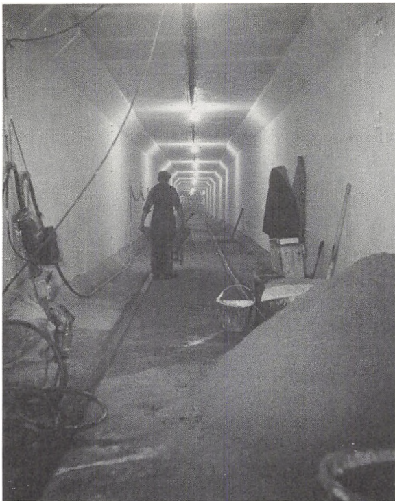
Den nye fjernvarmetunnel, Danmarks største, fra Christiansgade til svømmehallen, 650 meter lang, 3 meter høj og bred. En rutebil kan køre i tunnelen, hvis der ikke også skulle være fjernvarmerør. Billedet viser den første del af tunnelen fra Christiansgade til Regina-krydset, oktober 1953. (Foto: Lokalhistorisk Samling)
