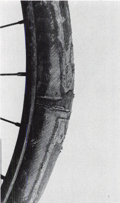
Detalje af det hjemmelavede dæk. Man kan tydeligt se, hvor dækket er vulkaniseret. (Foto: Flemming Rasmussen, Roskilde Museum).
