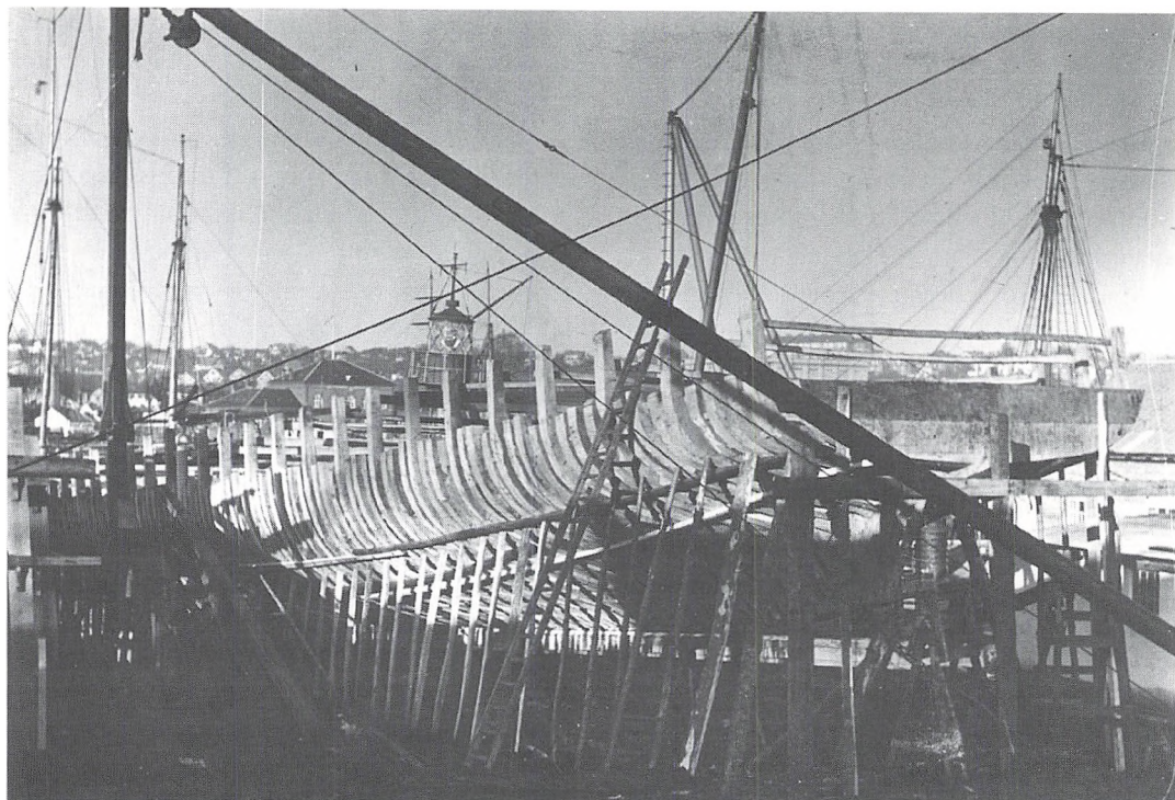
Den nye Vindebyfærge på bedding hos Ring-Andersen. Debatten om den nye færges bredde fortsatte gennem efteråret 1945. Færgen blev først påbegyndt i efteråret 1946 og afleveret året efter.
