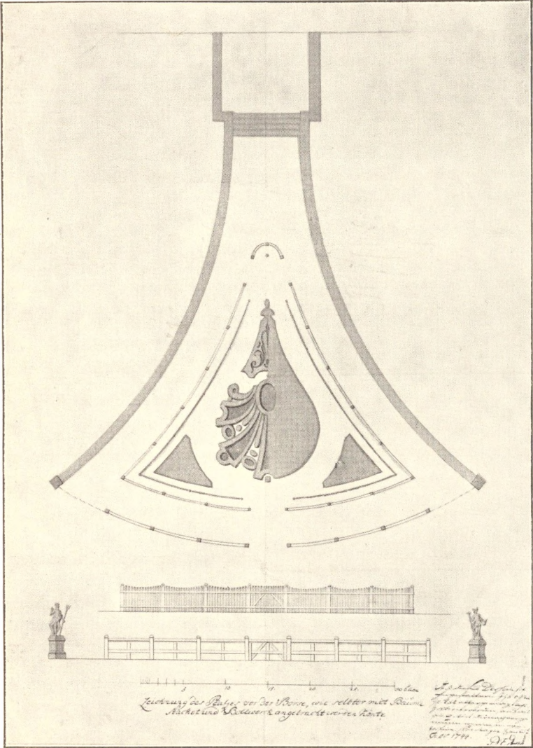
Forslag til Børsrampens Beplantning med Træer, samt Stakit og Bolværk. Eigtveds approberede Tegning, 1744.
