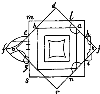
20. Konstruktion paa en Ottekant.
