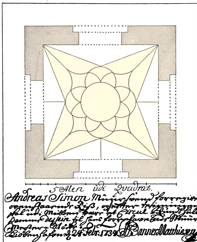
65. Gewelft at opmure til Mesterstykke 1734.
