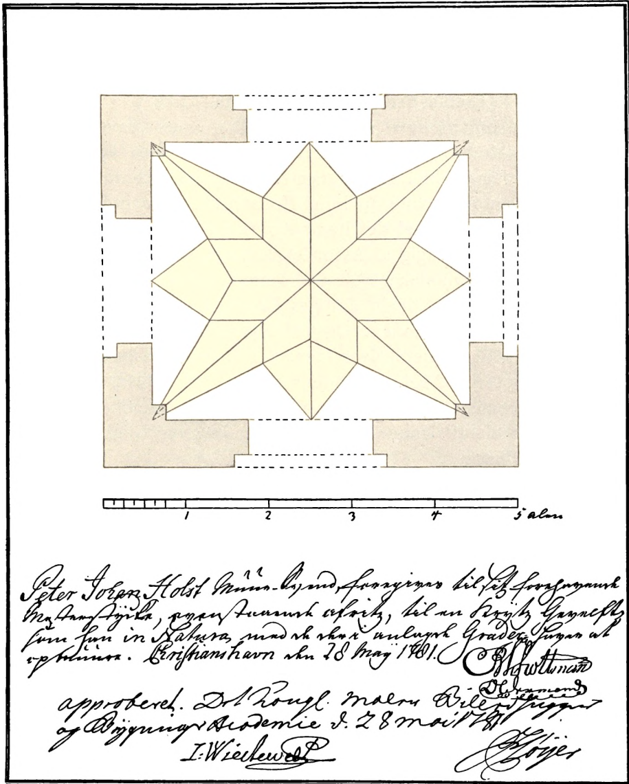
66. Gewelft at opmure til Mesterstykke 1781.
