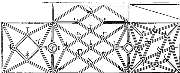
11. Hvælvingsplan med indskrevne Mærker.
