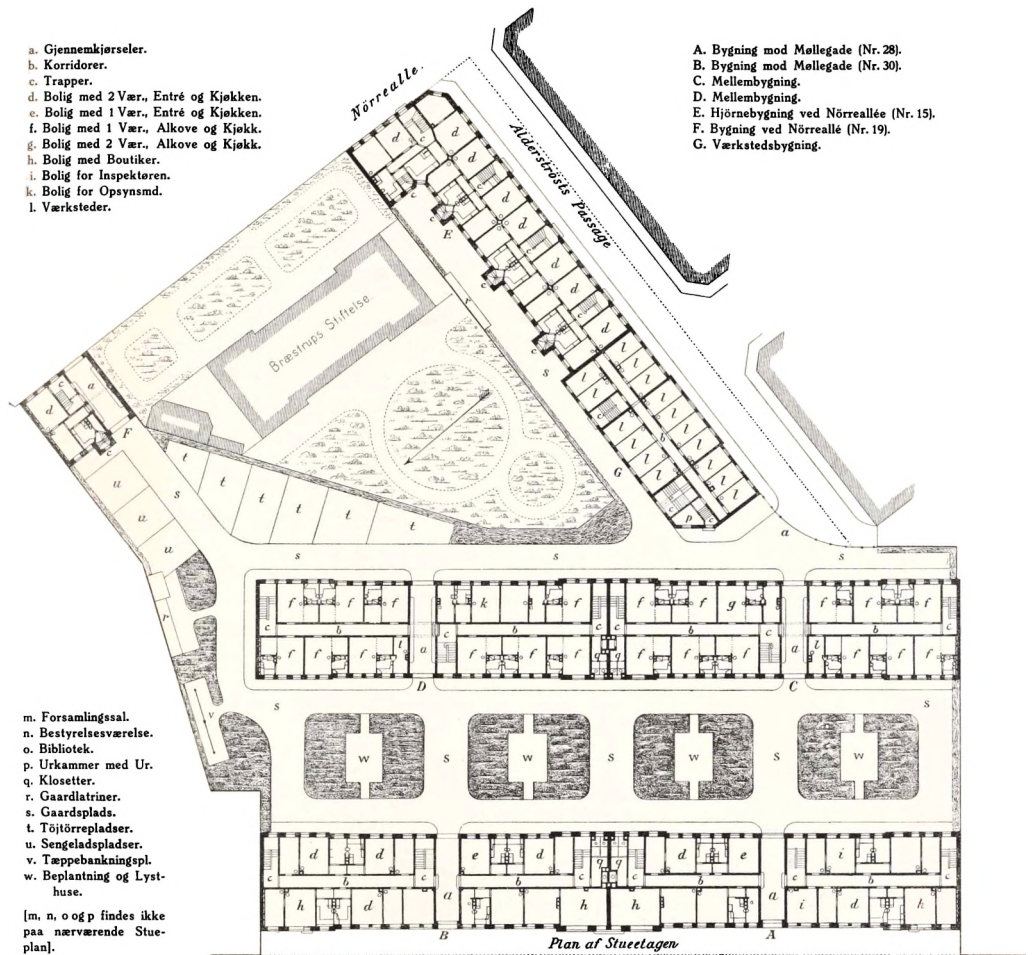
Plan af Stuelagen
