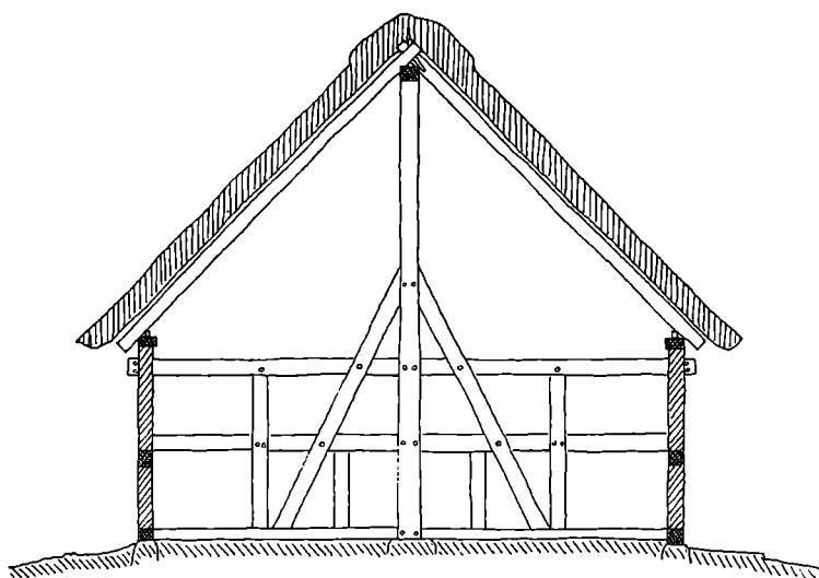
Tværsnit af en Gård fra Grimstrup (1723).
