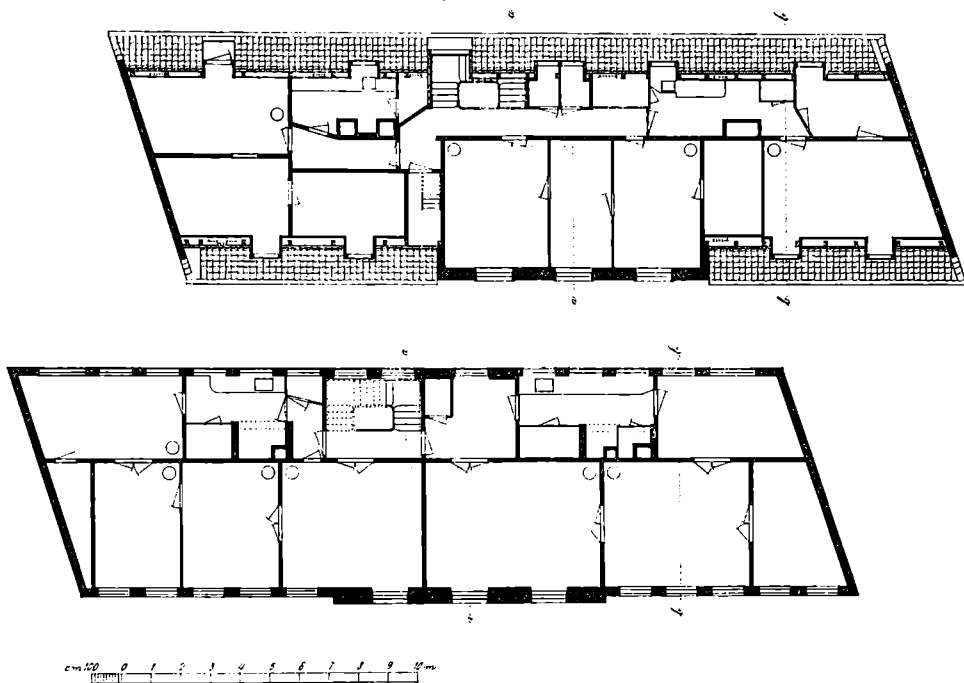
Frederiksberg Bredegade Nr. 26. Planer af 1. Sal og Tagetage.
