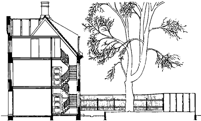
Frederiksberg Bredegade Nr. 26. Gaardfacade og Snit a-a.
