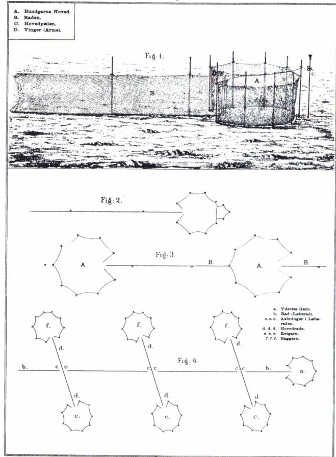
Bundgarn, tegning i C.F. Drechsel: Vore Saltvandsfiskerier, Kbhvn. 1890.
