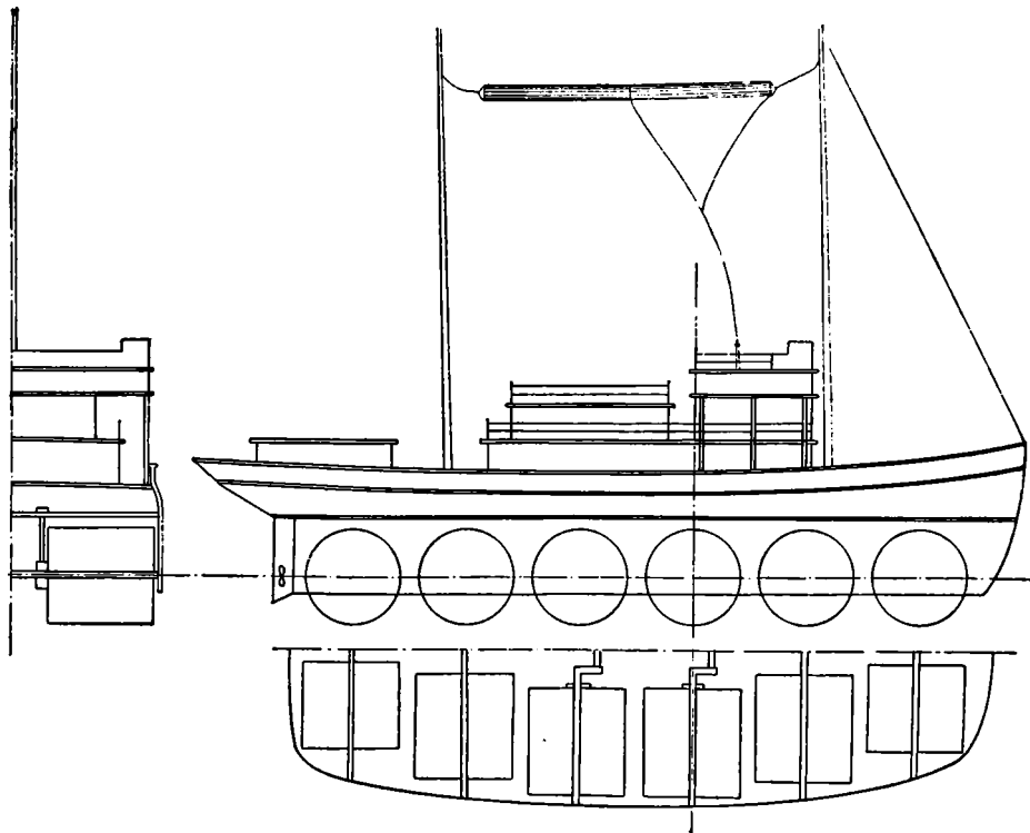
Tegningen af Et hurtigtgaaende Skib er udført af stud. polyt. Arne Fredborg paa Grundlag af Carl E. Simonsens Tegning fra 1896.
