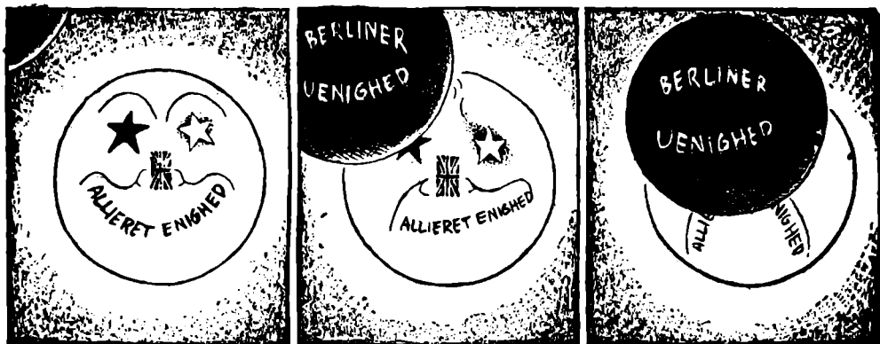
Solformørkelsens Faser.
