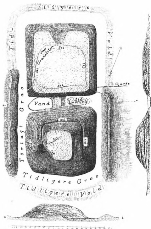
Fig. 3. I 1899 opmålte borgforskeren Peter Hauberg Hammersvold. Det kom der denne planskitse ud af.
