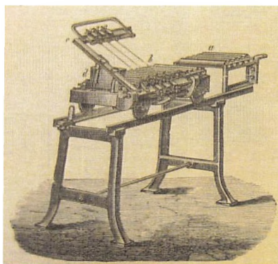
Universalskæ-reapparat (fra F. Borup: Teglværksindustri)
