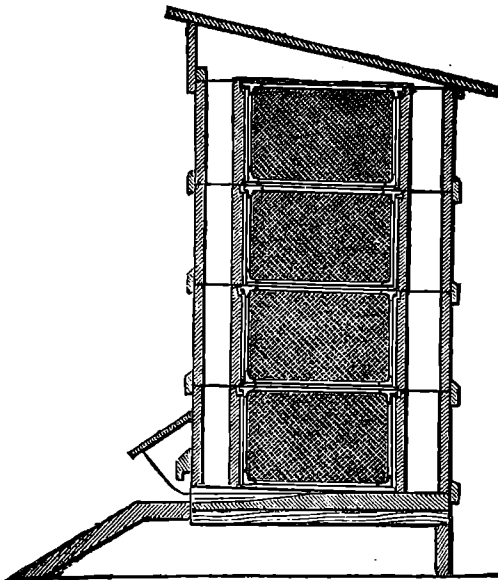
Fig. 4. Cowans Stabe, opstabelt.
