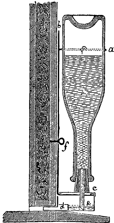
Fig. 15. Liedloff's Fodrer.
