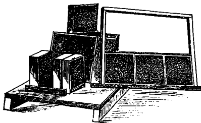
Fig. 10. Kærnestabe, aabent.
