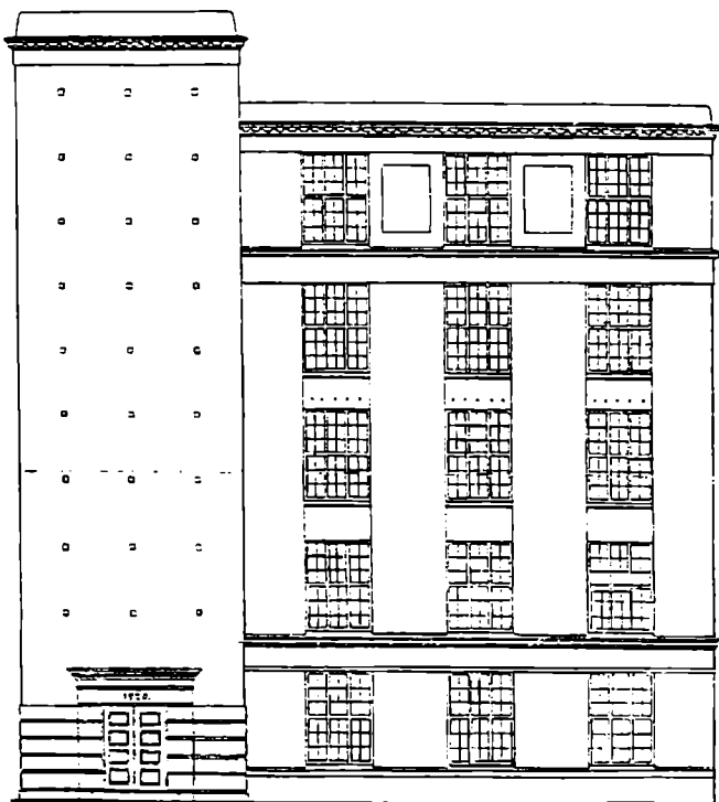
Reloucheret bygningstegning, der viser Brandts Klædefabriks såkaldte Pantheonfløj fra 1920, udført helt i jernbeton og beklædt med såkaldt bastardmørtel (Stadsarkivet).
