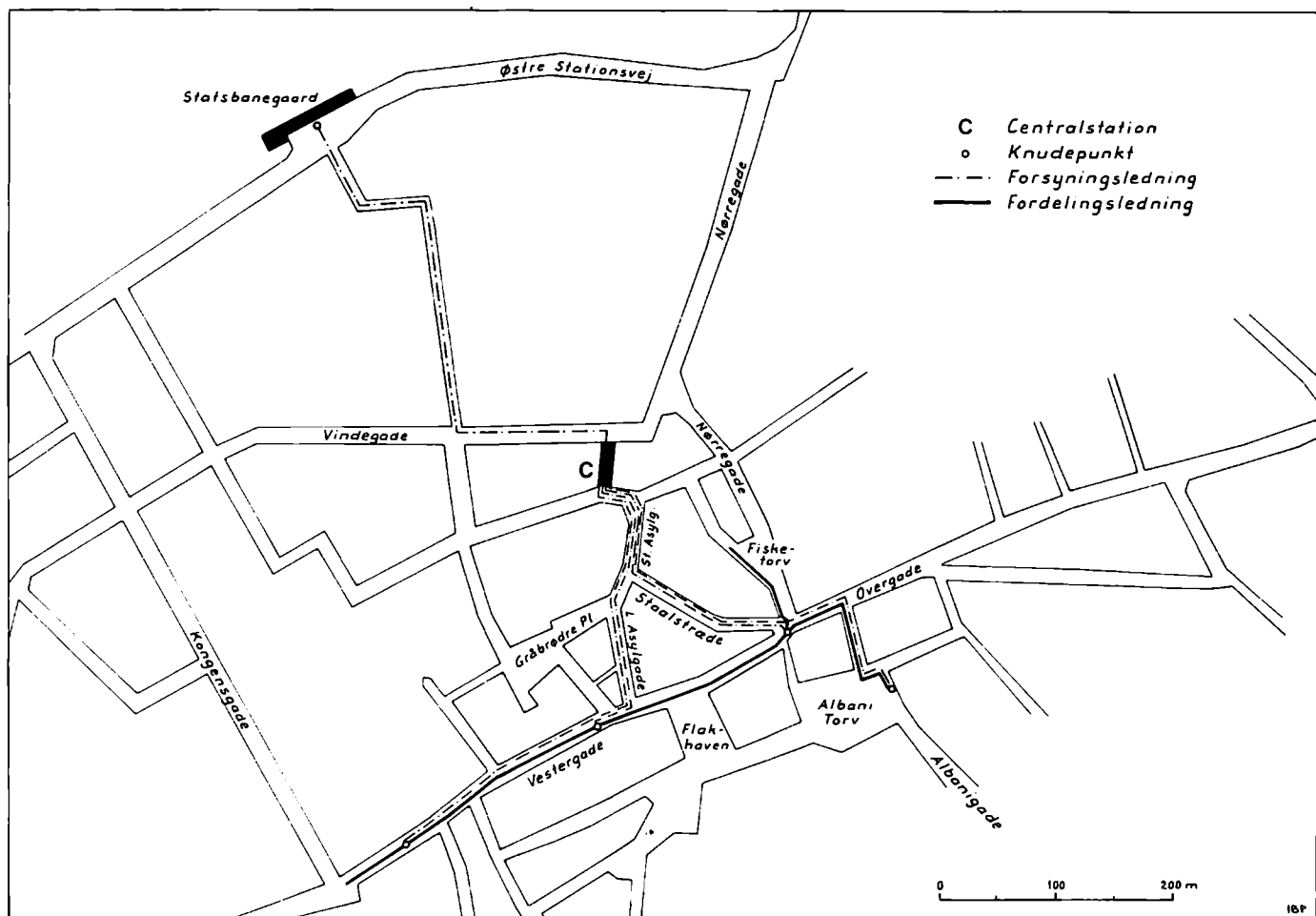
Planen for ledningsnettet, som Det danske Elektricitetskompagni præsenterede den for Odense byråd (Inger Bjerg Poulsen tegn.).
