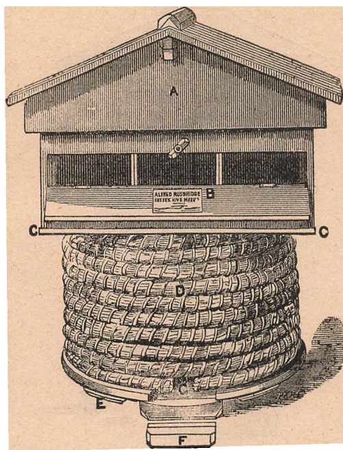
Fig. 1. Sukker Straa-Kube. A bevægeligt Tag. B Honningrum (med Støbben aaben), der kan rumme 21 Dellinger, hver med 2 Pund. C C Bundbrædt til Honningrummet. D Kuben. E Bundbrædt til Kuben. F Prop til Indskrænkning i Flydehullet G for at indskrænke det, naar Trættet er forbi.
