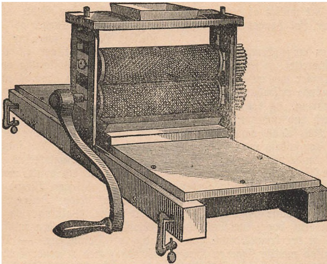
Fig. 8. Voks-Ark-Valse-Maskinen fra England.
