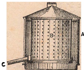
Fig. 51. Gersters Voks-Smelter. A Cylinderen. C Tuden, der fører det smeltede Voks fra Tallerkenen ud gennem Cylinderen B Vokskurven.
