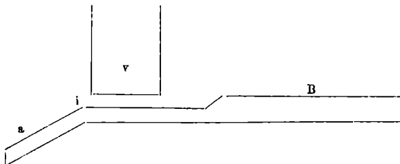
Fig. 33. Gennemsnit af et Bundbrædt med deri udskåret Indgang (i). B er Stadets Bund, a Flyvehæbræt, v den dobbelte Forvæg.
