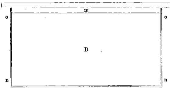
Fig. 42. Tør-Sukteramme til Fodring. D Døren; n n de to Stifter, der danne Hængslet; o o de to Stifter, der holde Døren fast; m den Ræbning, der giver Bierne Afgang til Sukkeret.
