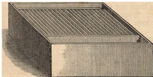
Fig. 47. Den kanadiske Fodrer. Gjennem Rummet foran og bagtil kunne Bierne gives Udgang. Alle det mellemste Rum's Bræder ere en halv Tomme lavere end Siderne. I det Num hæbes Foderet. Den dækkes med bitet Jærtraab-Løst og Tæpper.
