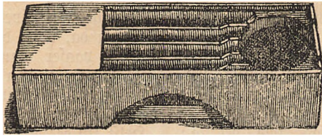
Fig. 42. Engelsk hurtig-Fodrer. Den hvide Udstilling paa Forsiden kan anvendes til Udgang for Bierne, Stillerrummene kunne da løbe helt igjennem; men det smalle forreste Rum maa da være afskilt helt fra det øvrige Rum, saa at det ikke fyldes med Sirup.
