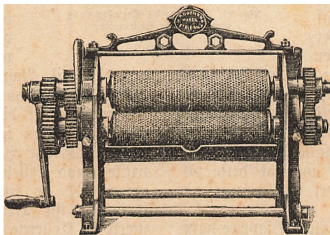
Fig. 24. Godman's Tablemølle med langsomt Drev og to Håndhaandtag.
