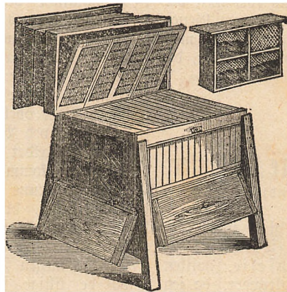
Fig. 5. Kilburn-Stadet, set bagfra og fra Venstre. Foroven til Højre ses en ubtaget Delings- Kamme.
