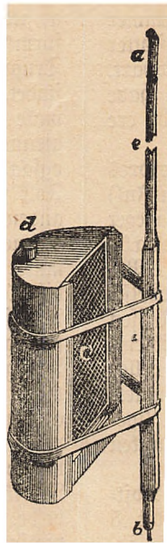
Fig. 46. Abbots Vidunder-Udslynger. a løst Haandtag, i hvilket Zornen ved e indfattes. Zornen ved b sættes ned i Gulvet. d er en Zub til Udtapning af Honning, e Traadnættet.
