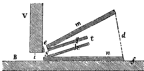
Fig. 31. Cheshires' Dronefælde. Gjennemsnit.
