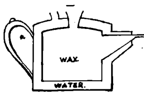
Fig. 24. Voks-Kobbe-Kande.
