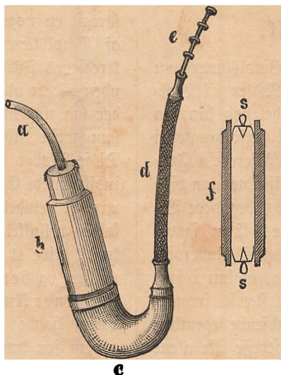
Fig. 4. Grønnings Pipibe. Til Højre ses et Gjenemsnit af Hovedet f.
