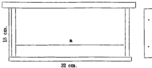
Fig. 13. Plan af en dobbelt dør i den øvre Yngelkasse D (se S. 39). Paa venstre Side ses den omtalte Dør, der paa Oversiden er beklædt med en Klædelibse, trykket fast paa sin Plads. Paa højre Side ses samme Dør med sine 2 smaa Pumpspliger færdig til at sættes fast. Ved a ses den dobbelte Hængning til midlertidig Befæstning af Mellemvæggen.
