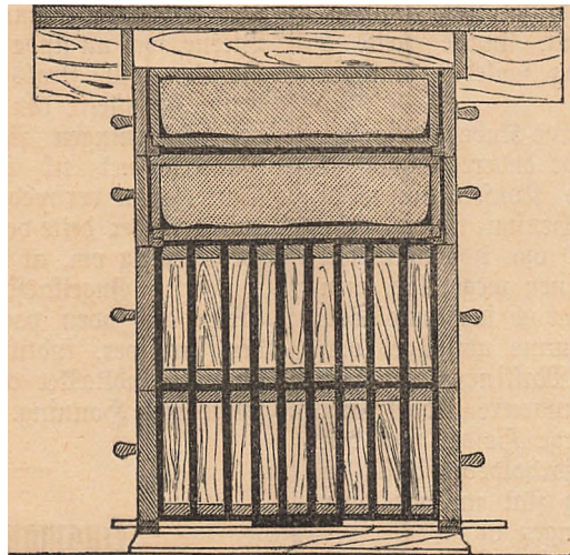
Fig. 7. Dahm's Magasin i \frac{1}{10} Størrelse (Gjennemsnit).
