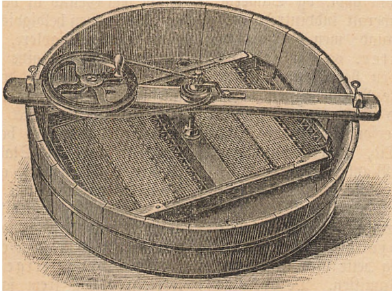
Fig. 3. Ubslynger med vandrette Tavler.
