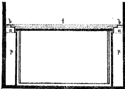
Fig. 34. Bivej over Tavlebærerne, l Tæppe, p Pakning.
