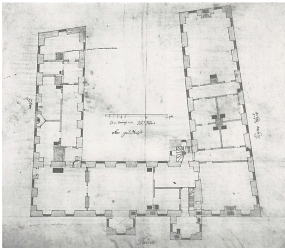
Tirsbæk, Hatting herred Vejle amt. J. G. Hödrichs plan af første sal med indtegnede ændringer.
