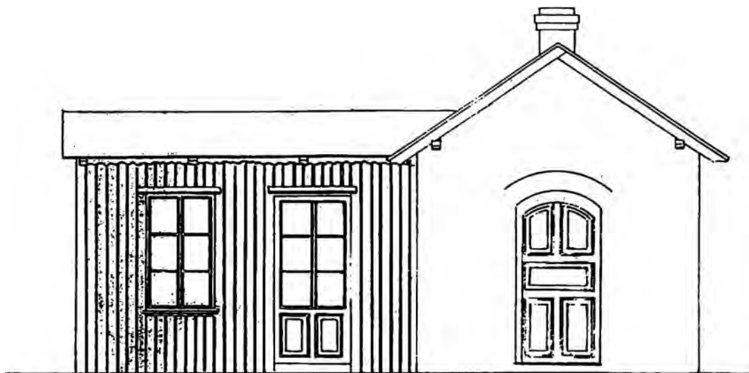
Styding Station bygget 1867. Tv. ventesalen bygget i træ og th. vogterhytte til materiel og brændsel. (Tegning fra DSB's arkiv).
