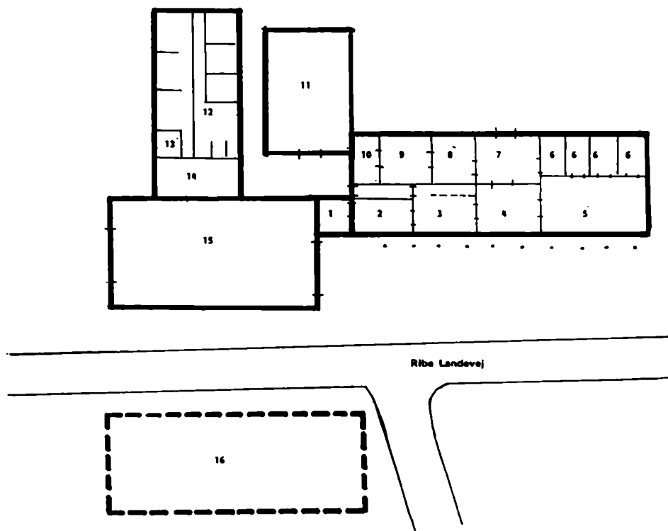
Grundriss af kroen, som den så ud inden branden i 1899 efter Didrik Thomsens beskrivelse. 1. gang. 2. forstue. 3. skænkestue. 4. krostue. 5. sal. 6. gæsteværelser. 7. havestue. 8. soveværelse. 9. køkken. 10. spisekammer. 11. natstald. 12. stalde. 13. "boskammer". 14. lade. 15. kørestald. 16. avlsbygning til 1880.
