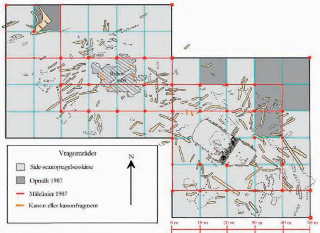
Oversigtsplan over DANNEBROGES vraglokalitet. Tegning J. Christoffersen 1988. Rentegning: Claus Rohden Olesen 2004.
