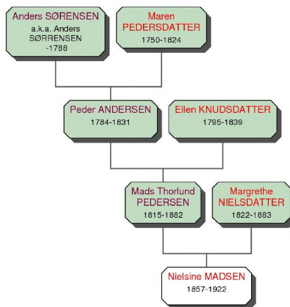
Figur 19: Stamtræ - Thorlund-slægten
