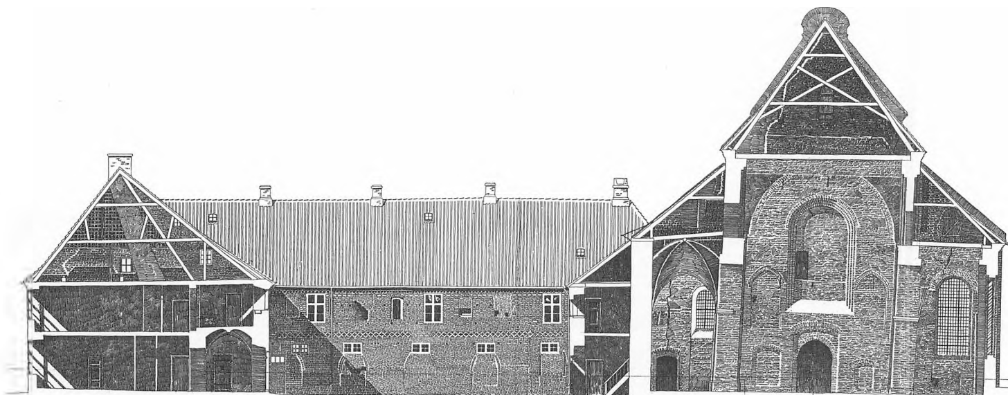
FIG. 22 Vestfløjens gårdfacade med snit gennem sydfløjen og kirken. 1 : 300. Målt af Axel Hansen 1918–20.
