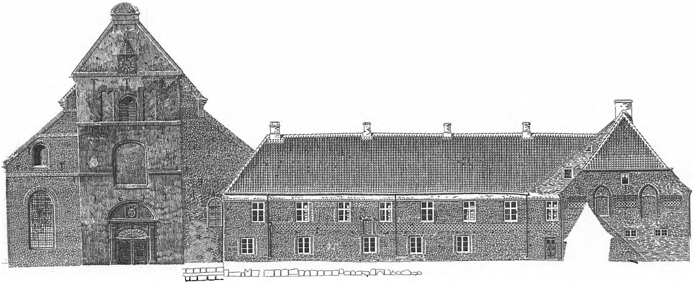
FIG. 23 Klostrets front mod vest. 1 : 300. Målt af Axel Hansen 1918–20.
