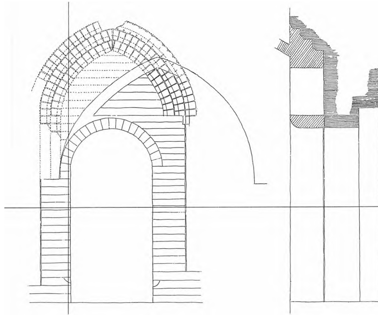
FIG. 14 Skt. Katharinæ kirke. Søndre sideskibs mur. Portal fra nordre korsgang. 1:50. Målt af Axel Hansen 1921.
