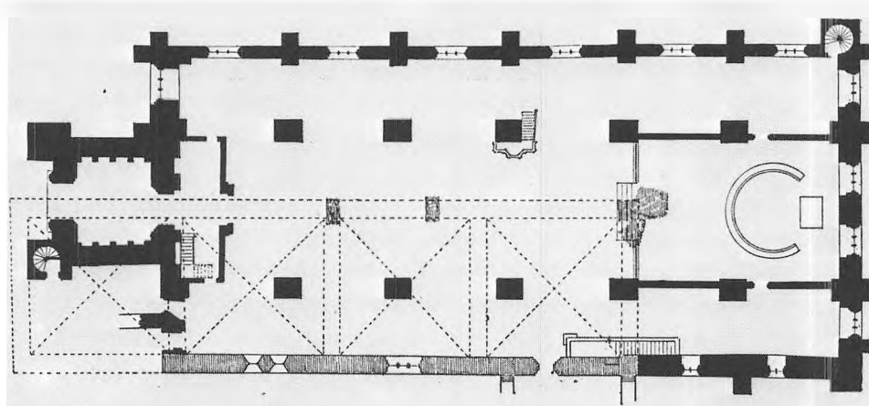
FIG. 11 Skt. Katharinæ kirke. Plan. Med stiplede linie er indtegnet den ældste kirke (nr. 1), med skravering er angivet bevaret murværk fra denne. Tegnet af Aa. Roussell(?). Trap V. udg. 1965.
