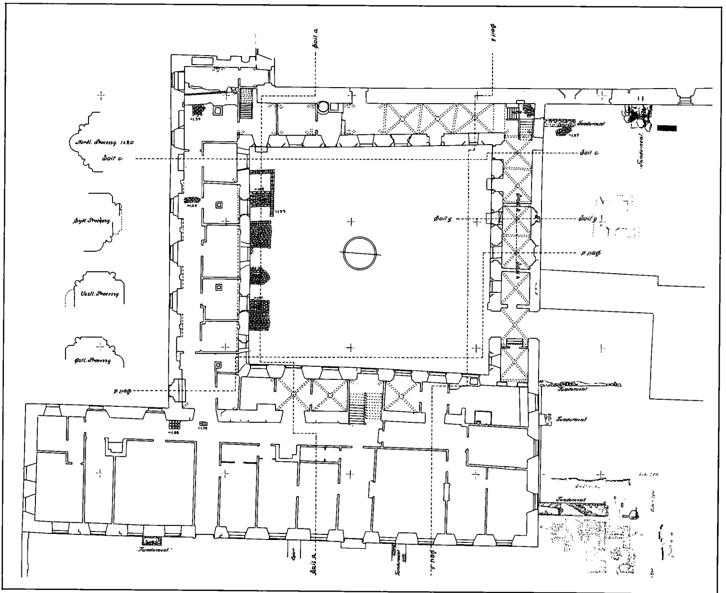
FIG. 15 Skt. Katharinæ kloster. Grundplan. 1:300. Målt af Axel Hansen 1918.
