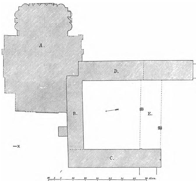
Situationsplan af Bjørnsholms bygninger og kirkeruin (Løffler).
